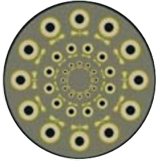
VB52754777 Ø 127 cm
